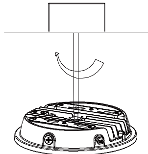
Conduit mount
